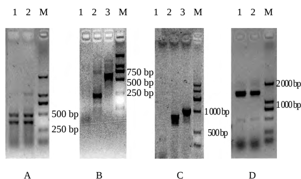
A-1, 2- FtF3'H 保守片段的扩增产物 B-1-3- FtF3'H 的 3'-RACE 的第 1-3 轮扩增产物 C-1-3- FtF3'H 的 5'-RACE 第 1-3 轮扩增产物 D-1, 2- FtF3'H ORF 的扩增产物 M-Marker
