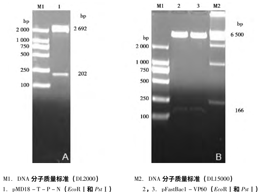
图3 pFastBac1 - DN 构建
