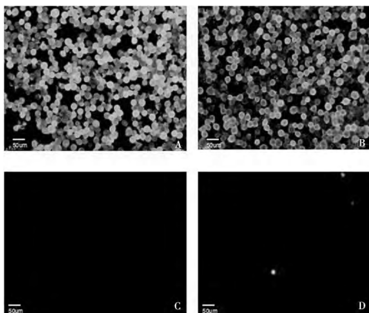
A. 感染重组病毒 rBac - VP60 的 Sf9 细胞 (阳性对照); B. 感染重组病毒 rBac - DN 的 Sf9 细胞; C. 正常细胞 (空白对照); D. 感染野生型杆状病毒的 Sf9 细胞 (阴性对照)
