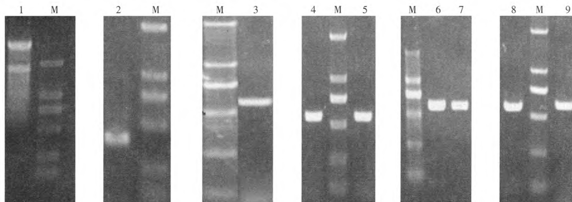
1: 叶片 RNA; 2: 3' RACE 扩增产物; 3: 5' RACE 扩增产物; 4, 5: PSAG1 ORF 扩增产物; 6, 7: PSAG2 ORF 扩增产物; 8, 9: 宜溪野生蕉基因组 DNA PSAG1 、 PSAG2 基因扩增产物; M: DL 2000 MAKER, 分子量从上到下分别是 2 000、1 000、750、500、250 和 100 bp。
