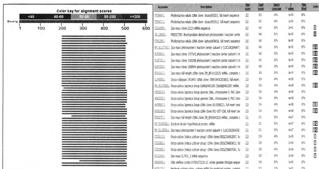
图 5 宜溪野生蕉 PSAG2 ORF 核酸序列 BLAST 结果
