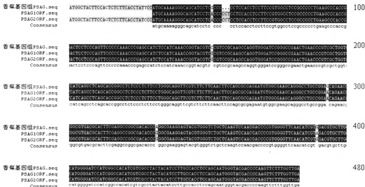
图 6 宜溪野生蕉 2 个 PSAG 成员的 ORF 序列与小果野蕉基因组的 PSAG 序列比对结果
