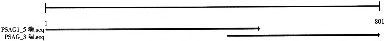
图 2 宦溪野生蕉 PSAG1 全长核酸序列拼接图
