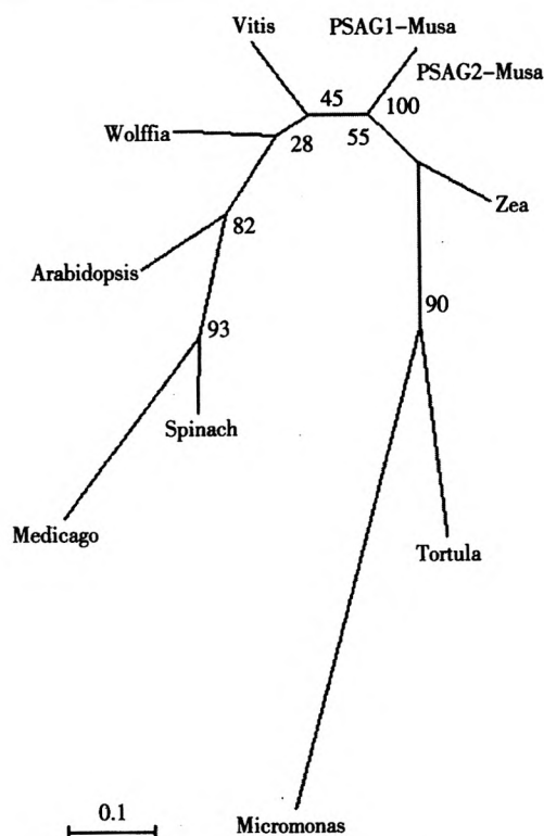
图 9 宜溪野生蕉 PSAG1 、 PSAG2 蛋白系统进化树
