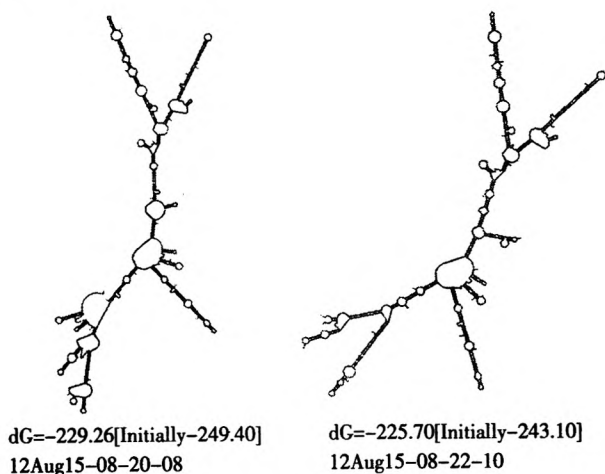
图 8 宜溪野生蕉 PSAG1 、 PSAG2 ORF 的二级结构分析
