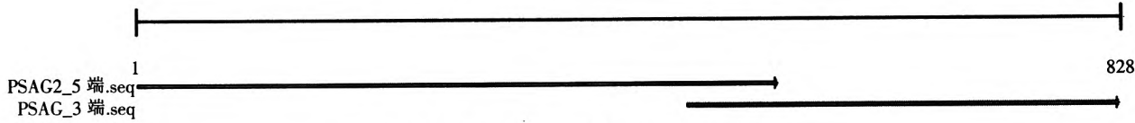
图 3 宦溪野生蕉 PSAG2 全长核酸序列拼接图
